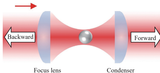
图 4 焦面干涉法原理示意图 [62]
