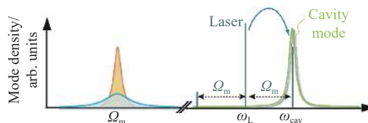
图 13 腔冷却原理示意图 [86]
