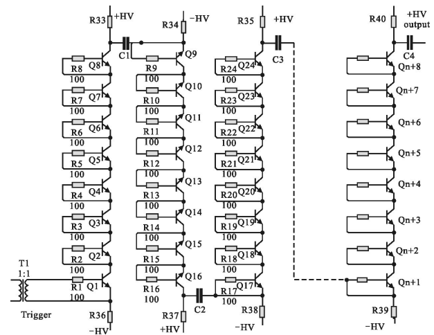
图 2 电路原理图
