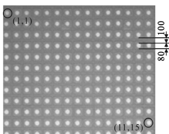
图 7 \mu\text{LED} 实际效果图
