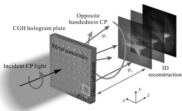
图 7 超颖表面纳米天线用作相位全息图进行三维计算全息记录和光学再现
