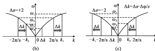
图 6 不同手性圆偏振光正入射下超颖表面对应的各衍射级次和 SPP 波矢匹配条件
