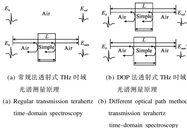
图 1 透射式 THz 时域光谱探测方法示意图
