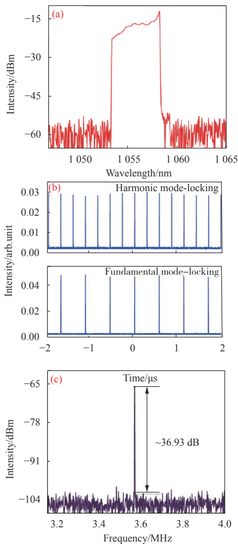
图 6 谐波锁模脉冲。(a) 光谱图;(b) 脉冲序列;(c) 射频频谱
