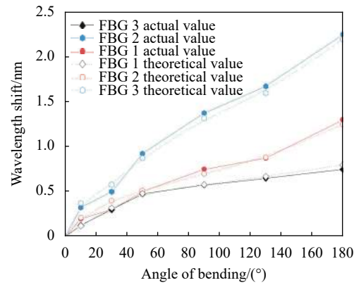
图 9 光栅中心波长漂移量与操作臂弯曲角度的关系
