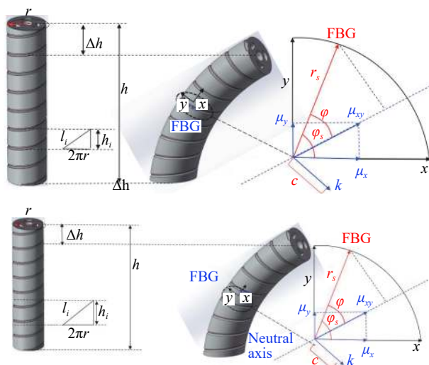
图 1 基于螺旋型光纤光栅的软体操作臂传感模型
