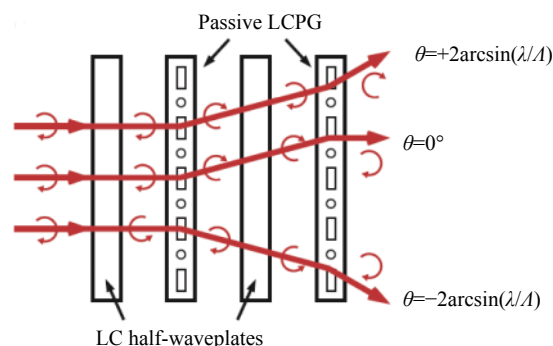
图 3 两个液晶可调半波片与两个 LCPG 组成的被动 LCPG 层
