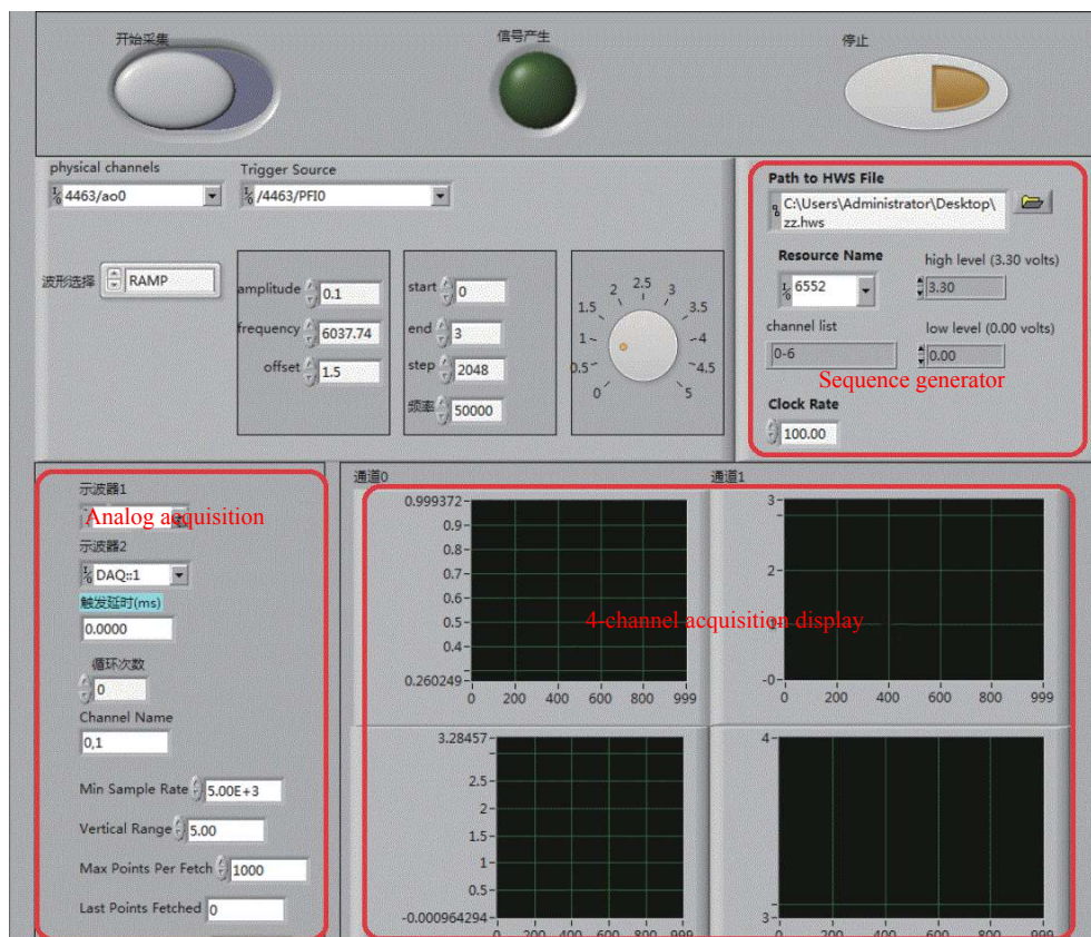
图 3 Labview 软件设计前面板及参数设置
