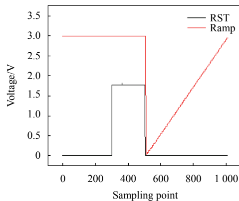
图 6 斜坡发生器固定时延
