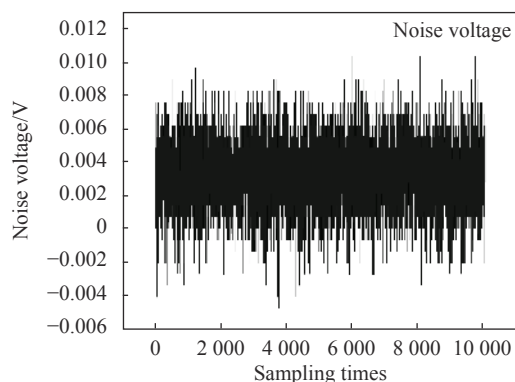
图 5 系统噪声测试
