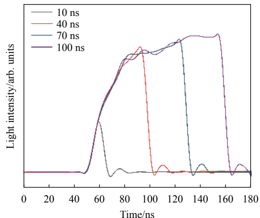
图 8 输出光波形
