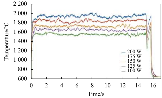
图 9 不同激光功率下熔池温度
