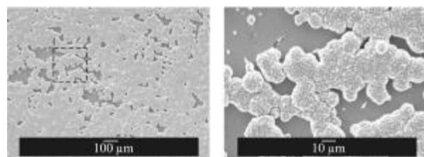
(e) 平均功率密度 400 kW/cm 2 (f) 表面形貌(e)的局部放大 (e) Average power density 400 kW/cm 2 (f) Local amplification of surface topography (e)
