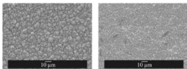
(c) 平均功率密度 300 kW/cm 2 (d) 平均功率密度 350 kW/cm 2 (c) Average power density 300 kW/cm 2 (d) Average power density 350 kW/cm 2
