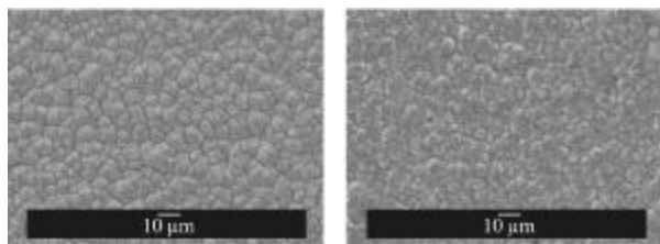
(a) 平均功率密度 100 kW/cm 2 (b) 平均功率密度 200 kW/cm 2 (a) Average power density 100 kW/cm 2 (b) Average power density 200 kW/cm 2
