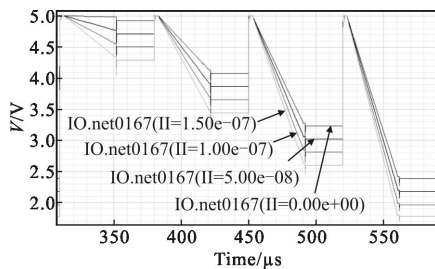
图 4 单元电路积分电压变化曲线 Fig.4 Integration waveform in unit cell
