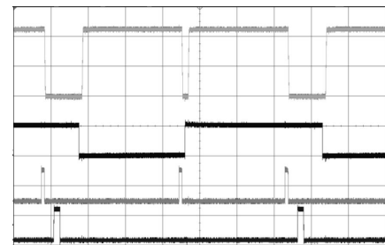
(b) 开启背景抑制
