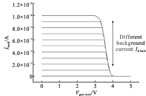
图 3 不同背景下背景抑制结构产生的背景减电流
