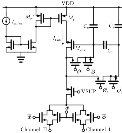
图 2 具有记忆功能的背景抑制结构
