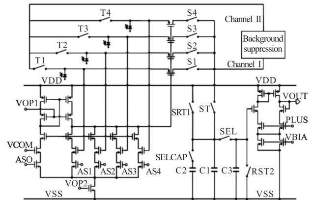
图1 共享型读出电路单元架构
