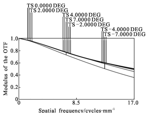
(a) -50 °C 时长波红外 MTF 曲线
