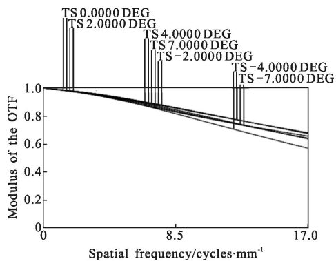
(c) 60^\circ\text{C} 时中波红外 MTF 曲线
