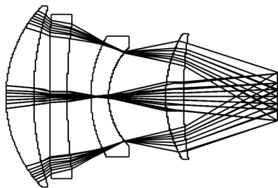
图 2 红外双波段光学系统光路图
