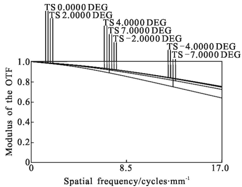
(a) -50^\circ\text{C} 时中波红外 MTF 曲线
