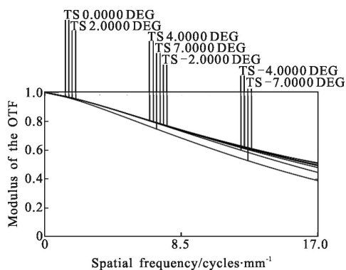
(b) 20 °C 时长波红外 MTF 曲线
