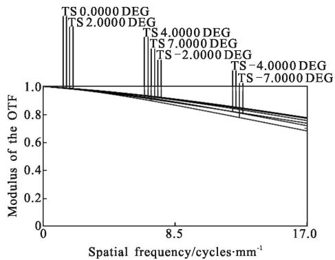
(b) 20^\circ\text{C} 时中波红外 MTF 曲线
