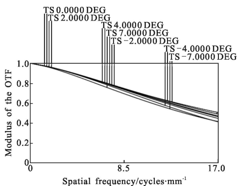
(c) 60 °C 时长波红外 MTF 曲线
