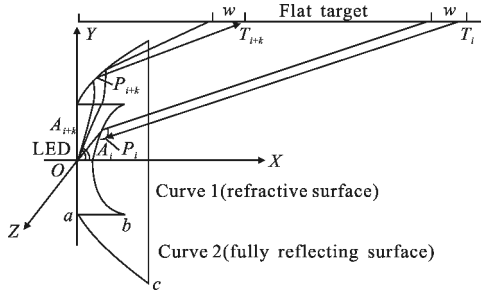
图 2 自由曲面透镜设计原理示意图
