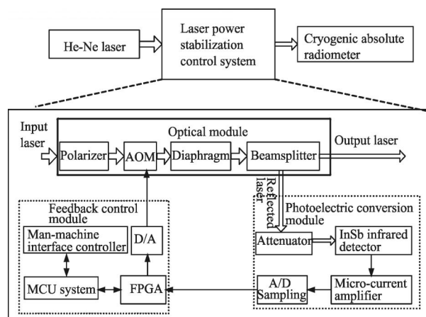
图 1 激光功率稳定系统结构
