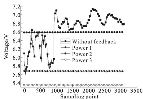
图 5 激光器不加反馈控制与加反馈控制后设定不同输出功率值
