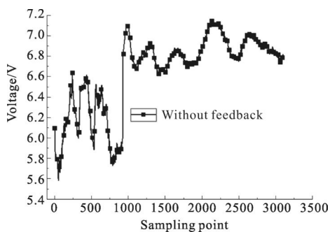
图 3 激光器不加反馈控制时输出功率曲线
