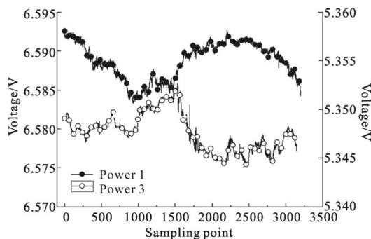
图 6 图 5 中 power 1 与 power 3 坐标放大后曲线
