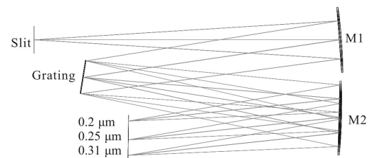
图 4 会聚照明光路图
