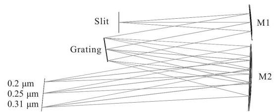
图 3 发散照明光路图
