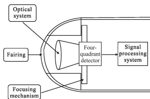
图 2 全捷联激光半主动制导寻的器结构组成图
