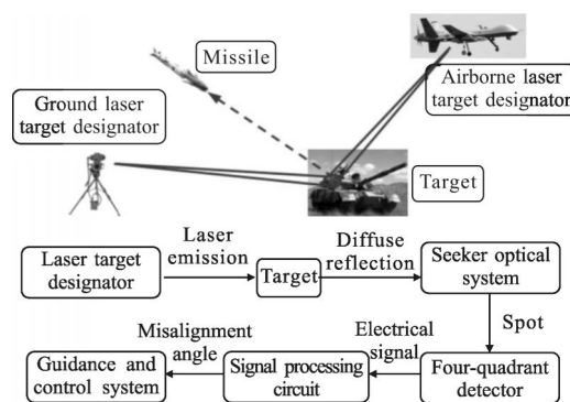
图 1 全捷联激光半主动制导武器系统工作原理图
