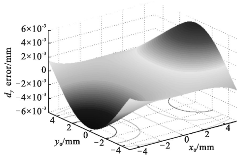
图 9 第二种放大模式引起的 d_y 误差
