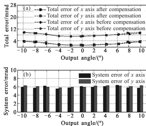
图 12 测角误差
