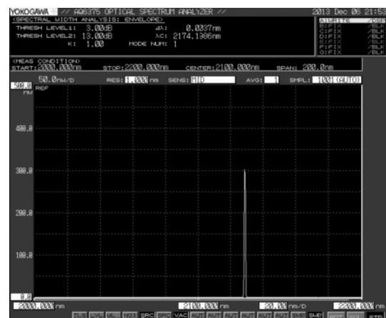
图 7 2.1 μm 激光波长示意图
