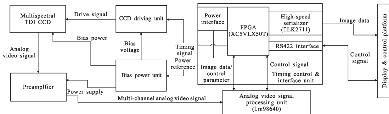
图 2 系统组成框图
