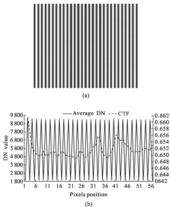
图 8 局部条纹图像与对应 DN 值及 CTF 值
