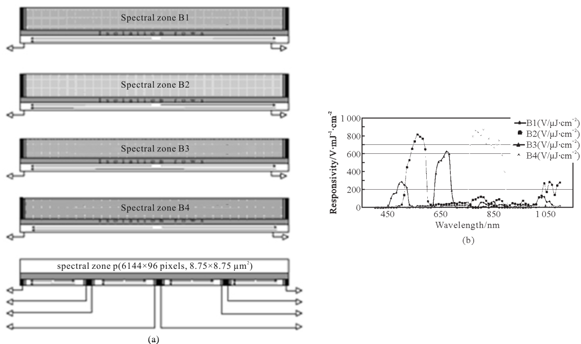
图 3 TDI CCD 结构组成(a)及多光谱谱段光谱响应曲线(b)
