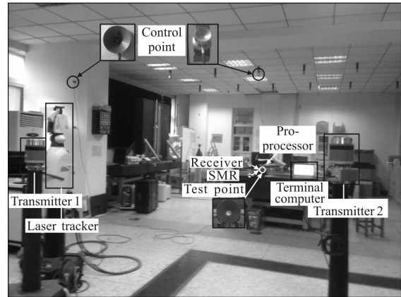
图 5 精度对比实验装置示意图
