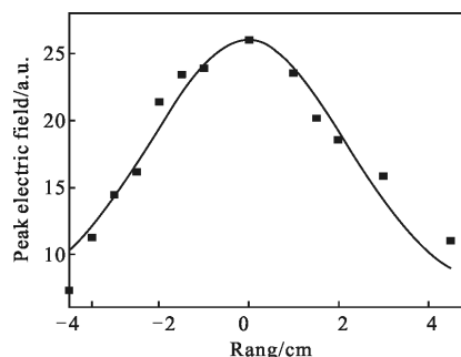
图 9 Z 轴方向场强分布高斯拟合图
