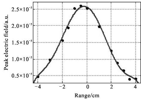
图 5 X 轴方向多项式拟合
