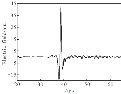
图 3 太赫兹波时域信号
