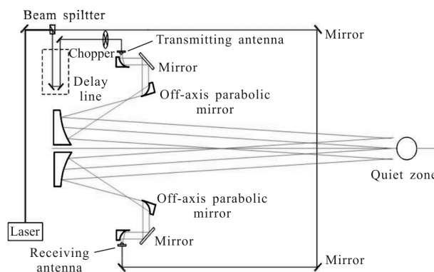
图 1 太赫兹时域光谱散射测量系统示意图
