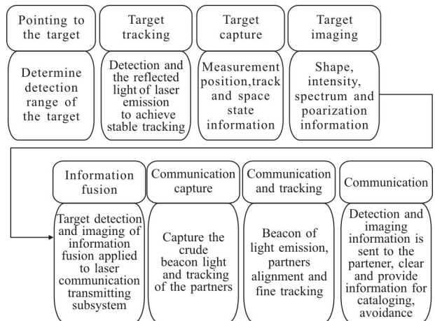
图 3 工作过程流程图
