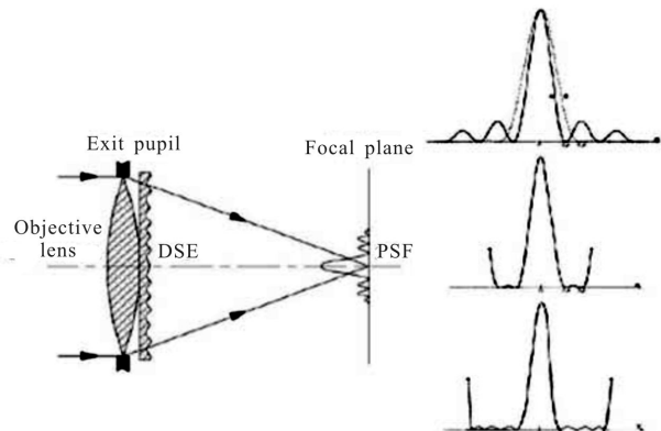
图 5 同心圆环调制出瞳函数实现光学超分辨
