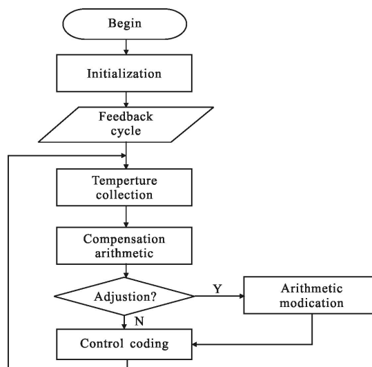
图 6 FPGA 控制流程图
