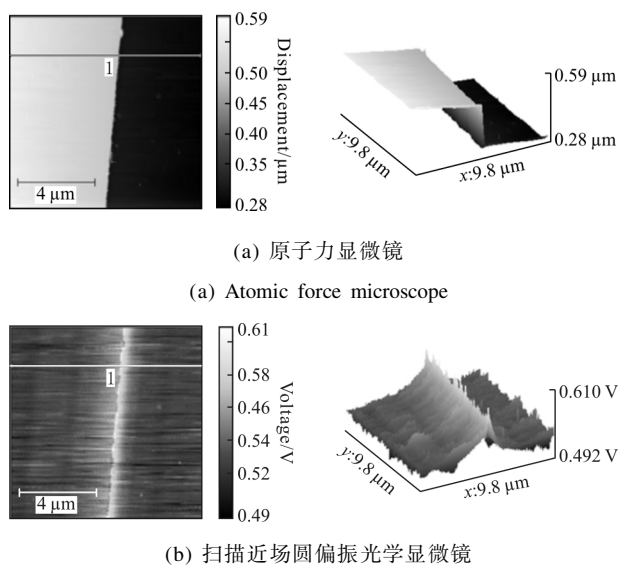
图 4 台阶样品的二维和三维形貌与近场光学图像
