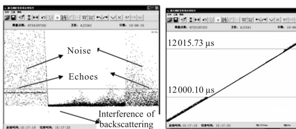
图 3 上海台高重复率 SLR 大气后向散射实验验证
