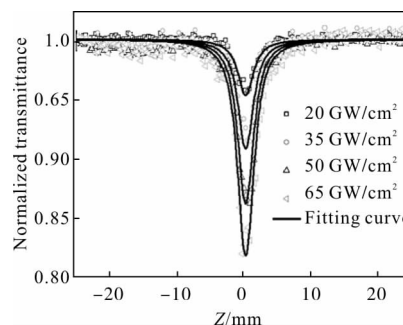
图 2 800 nm 飞秒激光激发的 RG665 开孔 Z 扫描实验结果
