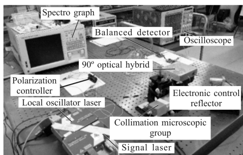
图 8 实验现场图
