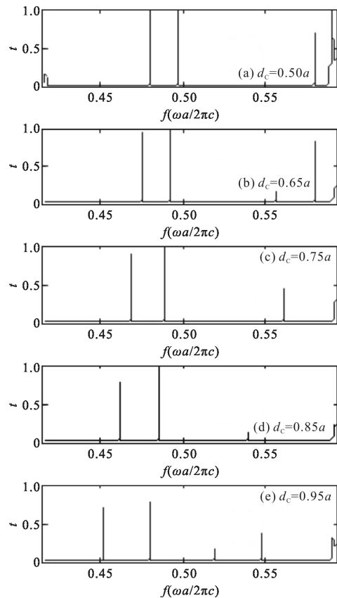
图 4 d_c 对 (TA)_5(PC)_2(TA)_5 透射谱的影响
