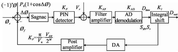
图 2 光纤陀螺的串扰模型
