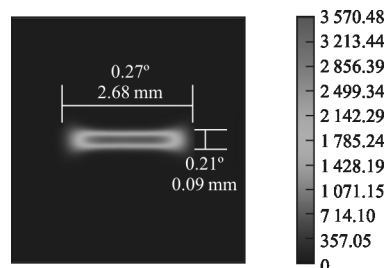
(d) 整形后的光斑
