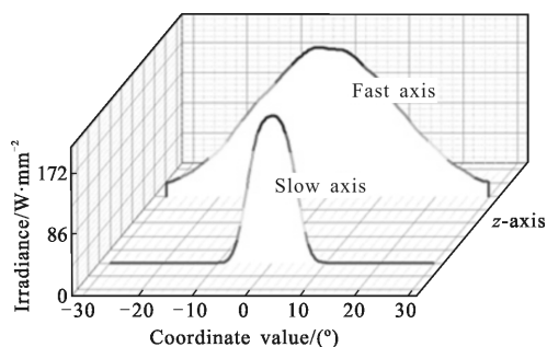
(a) 整形前的光发散角
