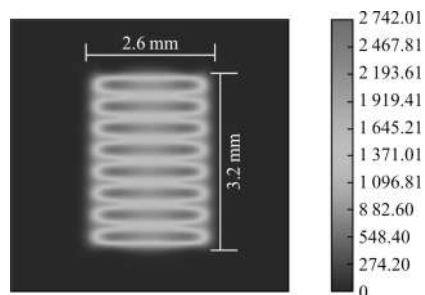
图 5 空间合束单元光斑图
