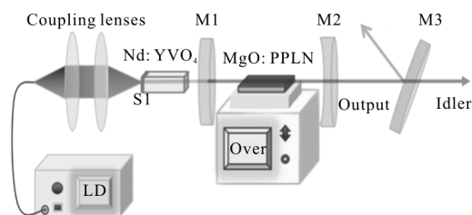
图 1 腔内抽运的 MgO:PPLN OPO 实验装置图 Fig.1 Schematic diagram of the intra-cavity MgO:PPLN OPO
