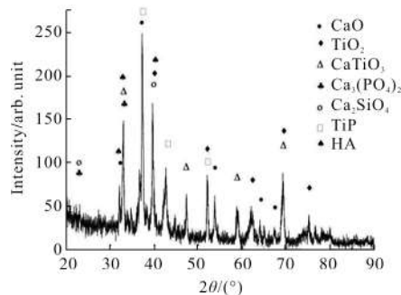
图 2 熔覆层的 X 射线衍射图谱
