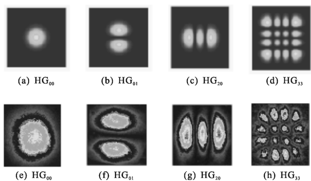
图 5 HG 光束的数值仿真与实验
