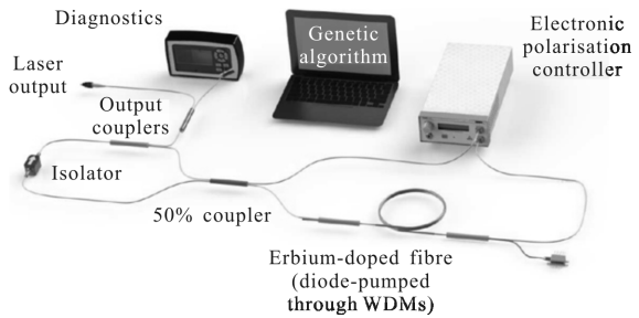
(b) 系统结构 (b) Experimental setup
