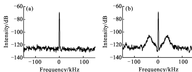
图 3 激光器锁模(a)和未锁模(b)状态时模间拍频信号
