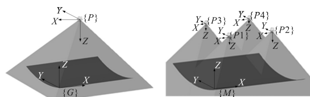
(a) 固定式投影仪站位 (b) 移动投影仪站位(4 站位)
