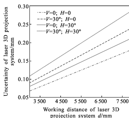
图 5 工作距离 d 与投影 uncertainty 关系
