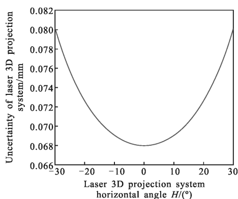
图 6 水平角 H 与投影不确定度关系
