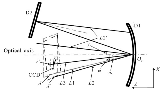
图 4 CCD 和理想反射镜发生偏转示意图
