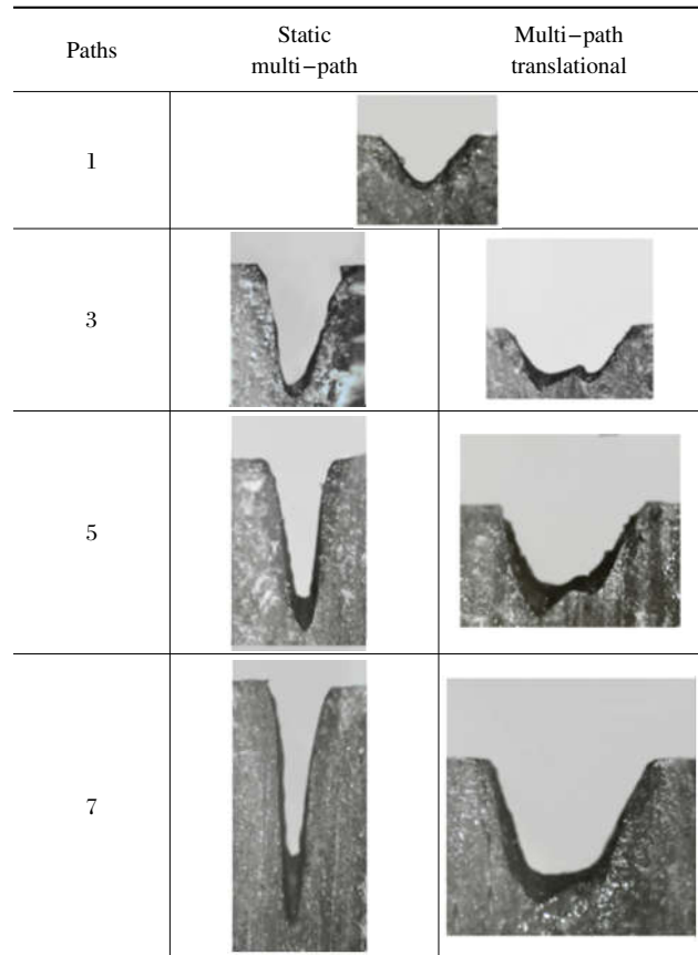
图 2 微通道的横截面对比图
