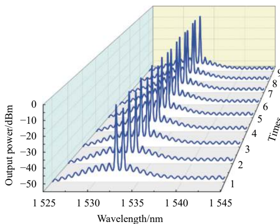
图 5 双波长状态稳定性测量
