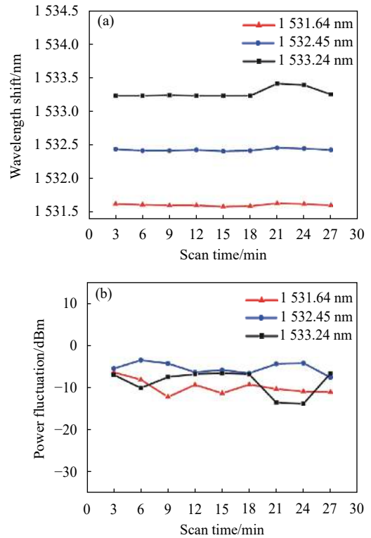
图 9 三波长在 27 min 内 (a) 波长漂移, (b) 功率波动测量
