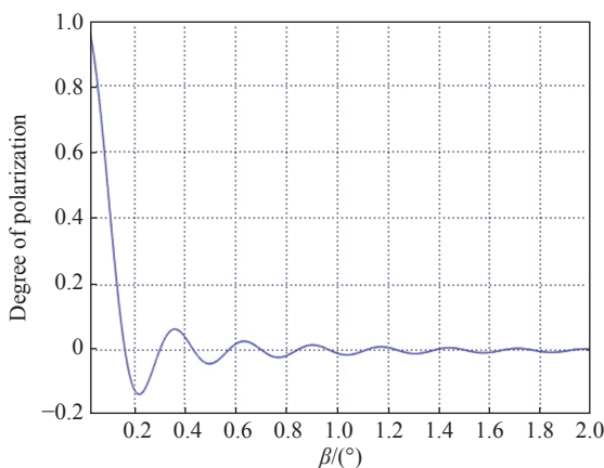
图 5 残余偏振度与楔角 \beta 关系
