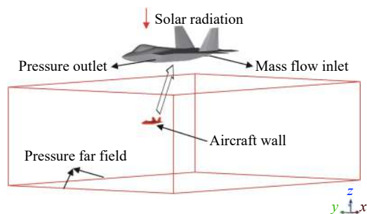
图 1 计算域和边界条件
