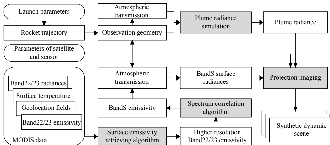
图 7 卫星观测火箭尾喷焰动态场景生成示意图
