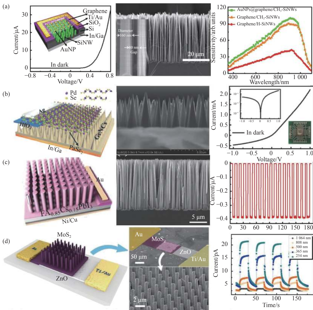
图 4 不同类型的纳米柱近红外光电探测器的结构及光电特性 [26-29] 。(a) 硅纳米线/金纳米颗粒/石墨烯探测器的 I-V 曲线和器件结构 [26] ; (b) 硅纳米线阵列/钙钛矿光电探测器的示意图 (横截面图和 850 nm 入射光零偏压下的时间响应曲线) [27] ; (c) PbSe 2 /GeNcs 阵列异质结光电探测器的示意图 (锗纳米锥阵列的横截面 SEM 图和 I-V 曲线图) [28] ; (d) ZnO/MoS 2 光电探测器的结构示意图 (SEM 图和时间-电流响应) [29]
