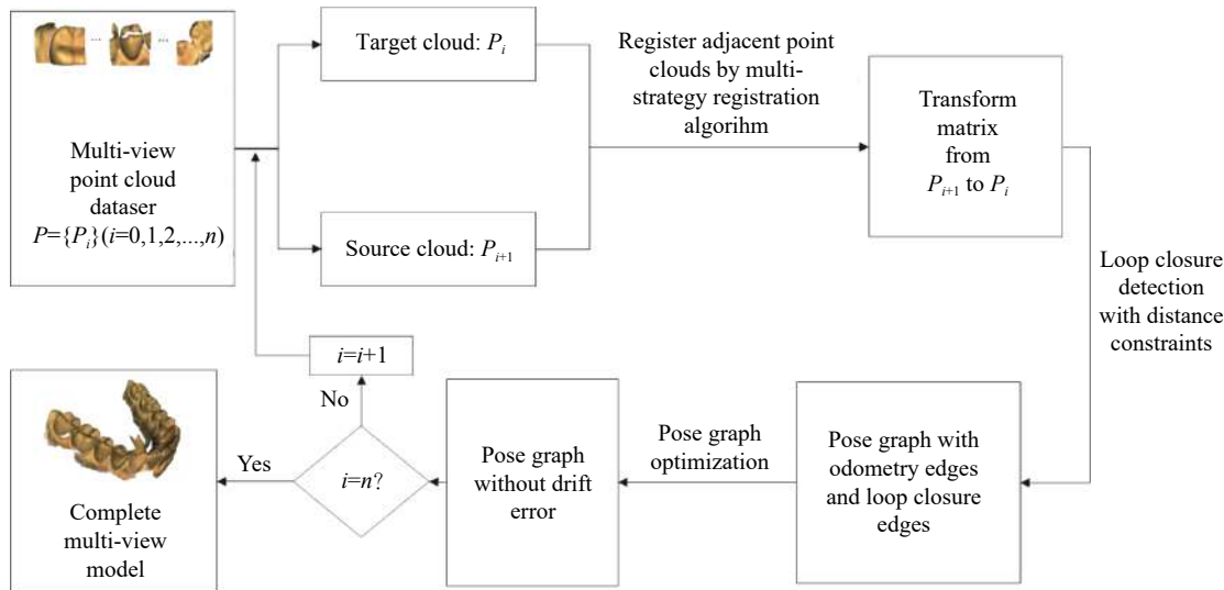
图 1 文中算法流程图
