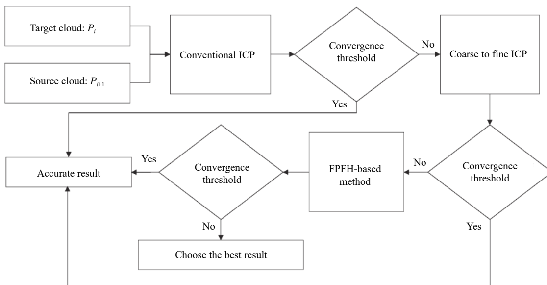
图 2 多策略融合配准算法流程图
