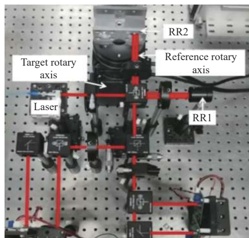
图 7 实验装置图
