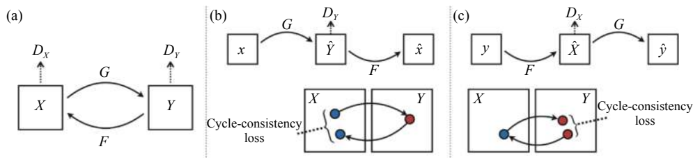
图 5 CycleGAN 的结构 [59] 。(a) 两个生成器循环生成图像; (b) X 域图像的循环重建过程; (c) Y 域图像的循环重建过程
