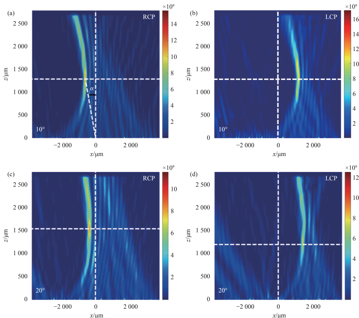
图 4 当 RCP 光以 10^\circ (a) 和 20^\circ (c) 分别入射时聚焦场的强度分布; 当 LCP 光以 10^\circ (b) 和 20^\circ (d) 分别入射时聚焦场的强度分布
