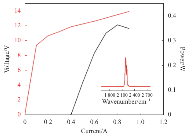
图 8 室温连续模式下的 L-I-V 和光谱
