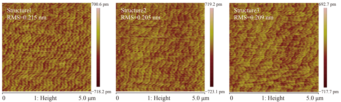
图 2 三种不同掺杂浓度样品的 AFM ( 5\ \mu\text{m}\times 5\ \mu\text{m} ) 测试结果图
