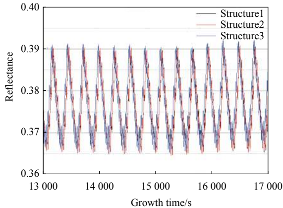
图 1 三种不同掺杂浓度样品的反射率曲线监控
