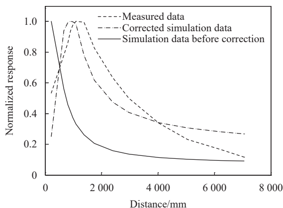
图 10 归一化激光雷达响应曲线
