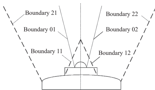
图 4 同轴激光雷达发射视场和接收视场
