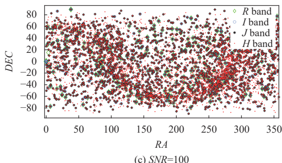
图 5 采用不同光学响应波段探测恒星分布图
