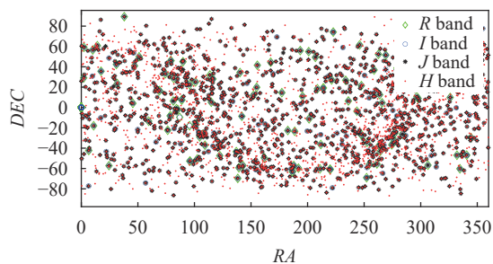
(b) SNR=50
